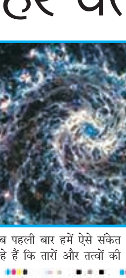
मात्रा के बीच का यह संबंध प्रारंभिक आकाशगंगाओं के लिए लागू नहीं होता है। इसका कारण संभवतः यह है कि ये आकाशगंगाएँ अभी बनने की प्रक्रिया में हैं, और उन्हें अभी तक भारी तत्वों को बनाने का समय नहीं मिला है।
